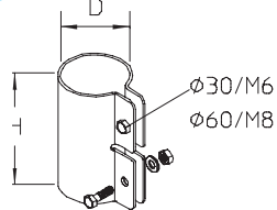
SRML Зажимная муфта, с перфорацией
